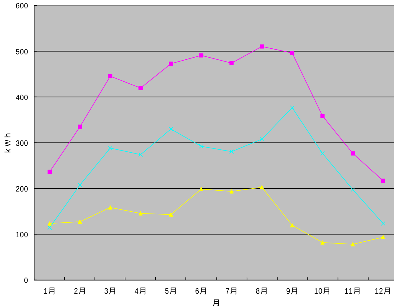
太陽光発電2002年実績値グラフ
