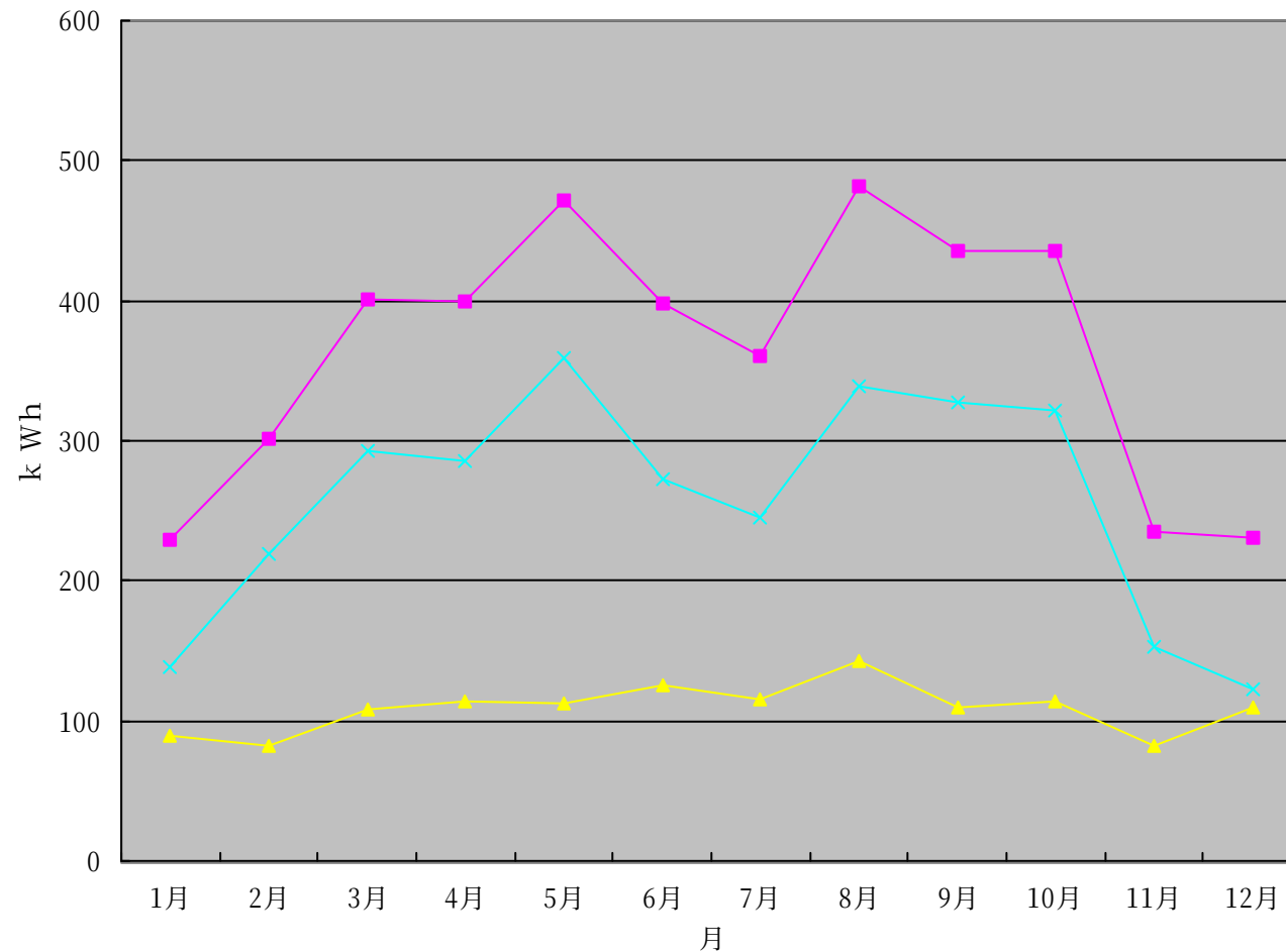
太陽光発電 2003 年実績値グラフ
