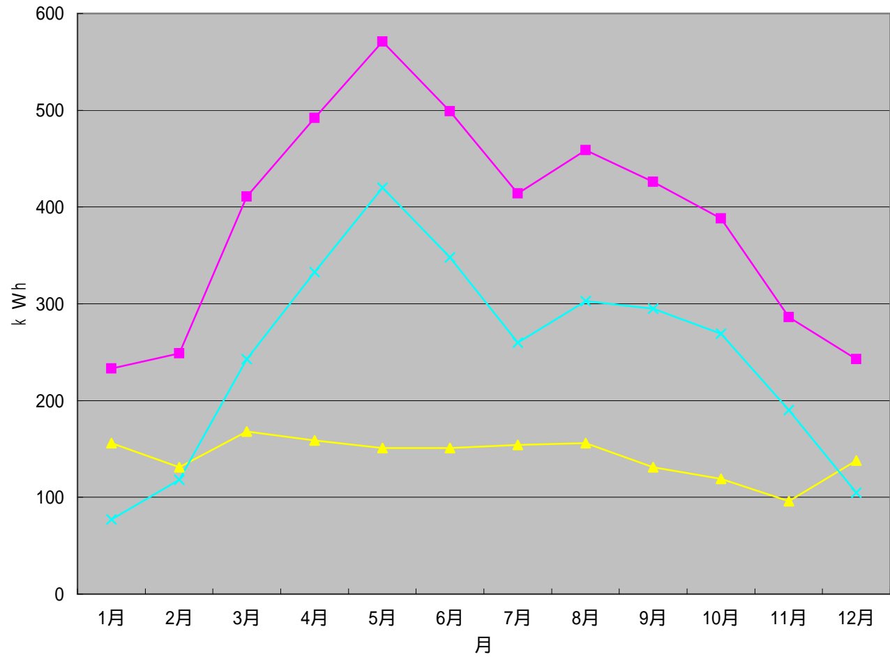
太陽光発電2005年実績値グラフ
